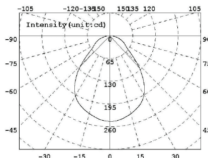
Intensity data:(deg , cd) C0-180
